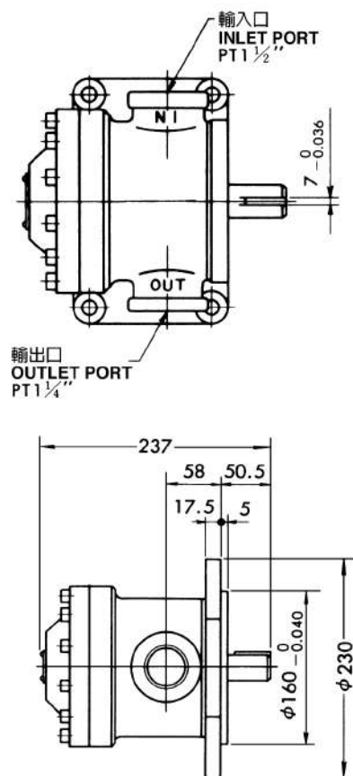
150T 法蘭式 Flange Type
