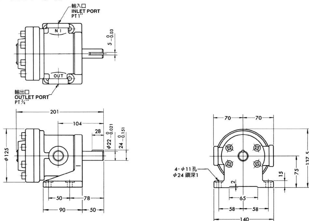
50T 腳座式 Lug Type
